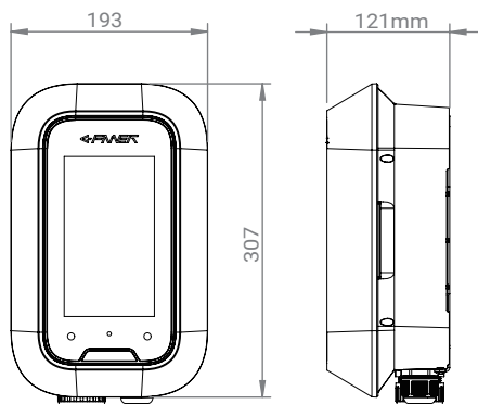
尺寸圖, 單位: mm
