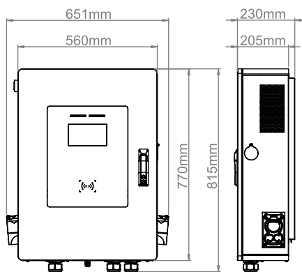
• 60 kW 尺寸圖 (單位mm)
