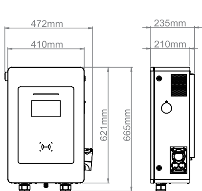
• 30 kW 尺寸圖 (單位mm)
